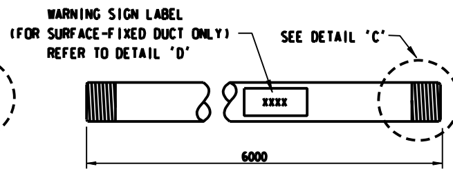
ELEVATION (G.I.)
